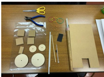
【実技研修】輪ゴム動力車
