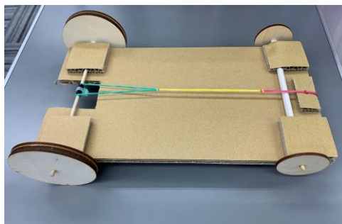
【実技研修】輪ゴム動力車
